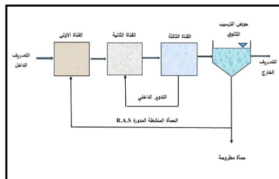
الشكل (2-b) مخطط أنسيابي في نظام القنوات الدائرية المتركزة (Orbal)
