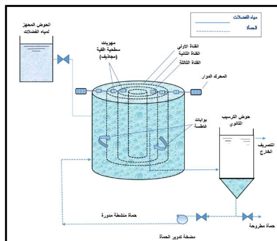
شكل (3) مخطط توضيحي لنظام القنوات الدائرية المتركزة (Orbal)
