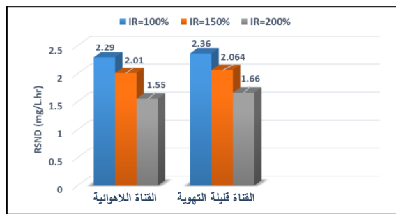
الشكل (8) معدل النتجة وعكس النتجة المتزامنة (RSND) في القناتين الخارجية والوسطية مع نسب التدوير الداخلي المختلفة عند نسبة تدوير خارجي (80%)
